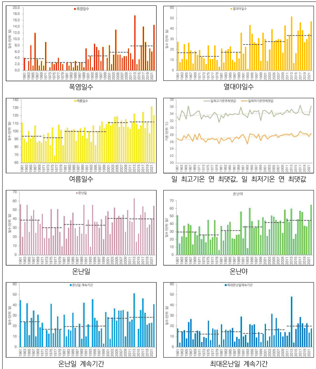
[그림 2-4-4] 고온 극한기후지수의 변화 (1961년~2022년)
