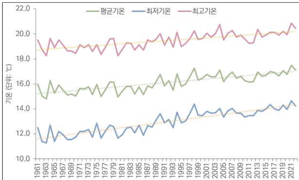
[그림 2-4-1] 과거 62년간 연평균 최고, 평균, 최저기온의 변화 (1961년~2022년)
