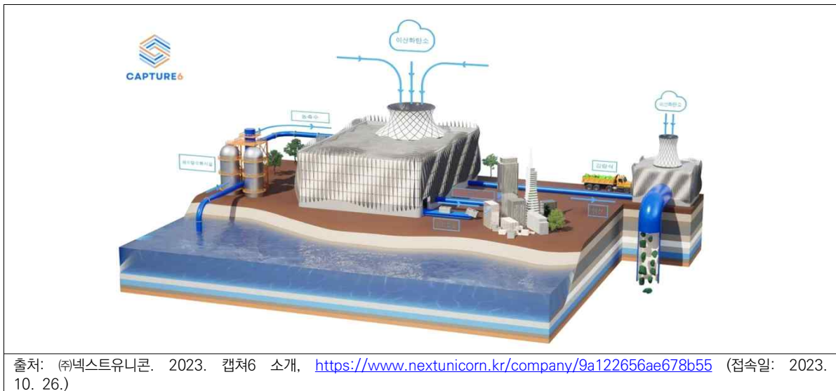
[그림 2-3-10] 습식 탄소포집 시설
