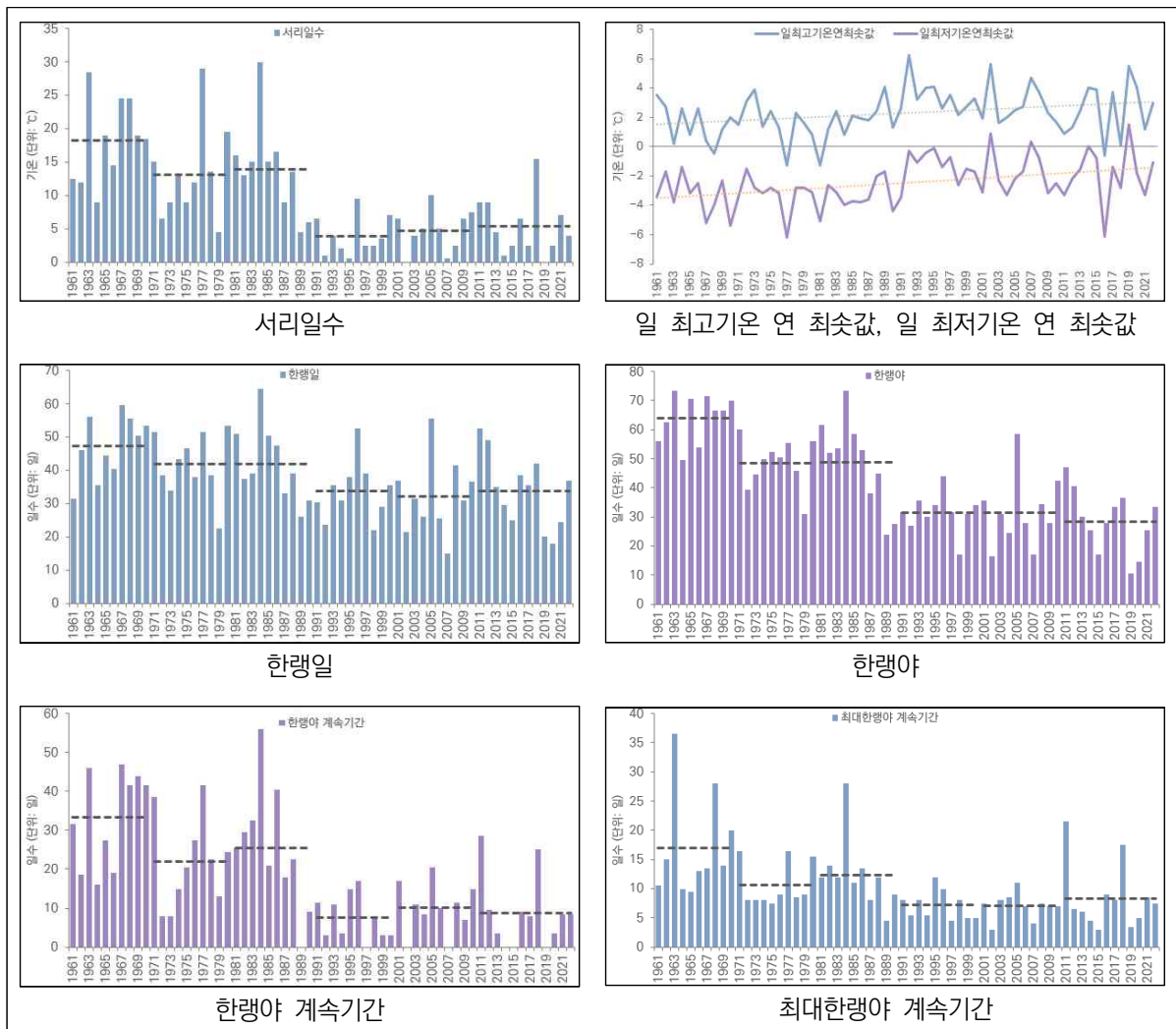
[그림 2-4-5] 저온 극한기후지수의 변화 (1961년~2022년)
