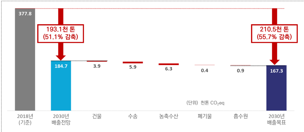
[그림 42] 2030년 온실가스 부문별 감축경로
