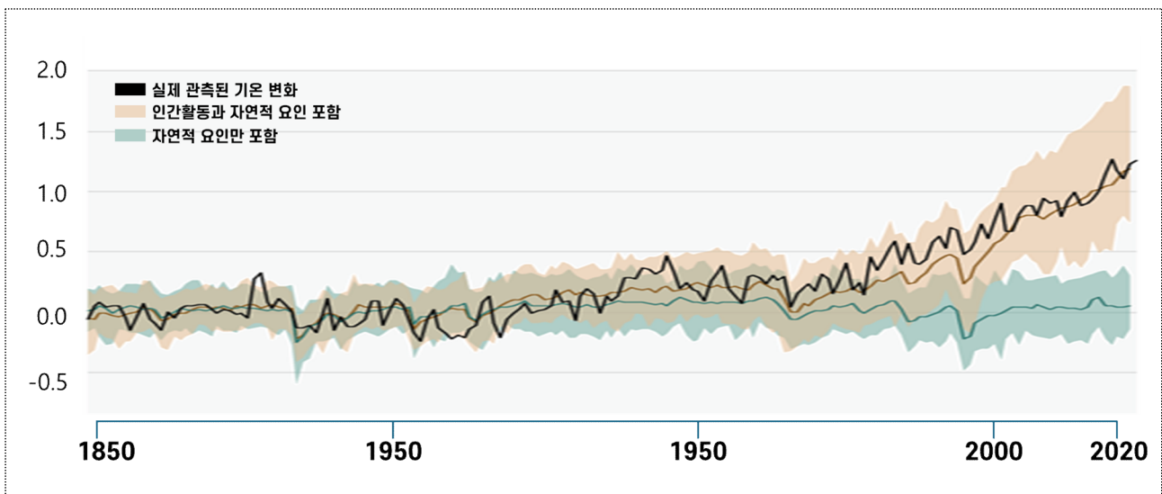
[그림 1] 전 지구 지표면 온도 변화
