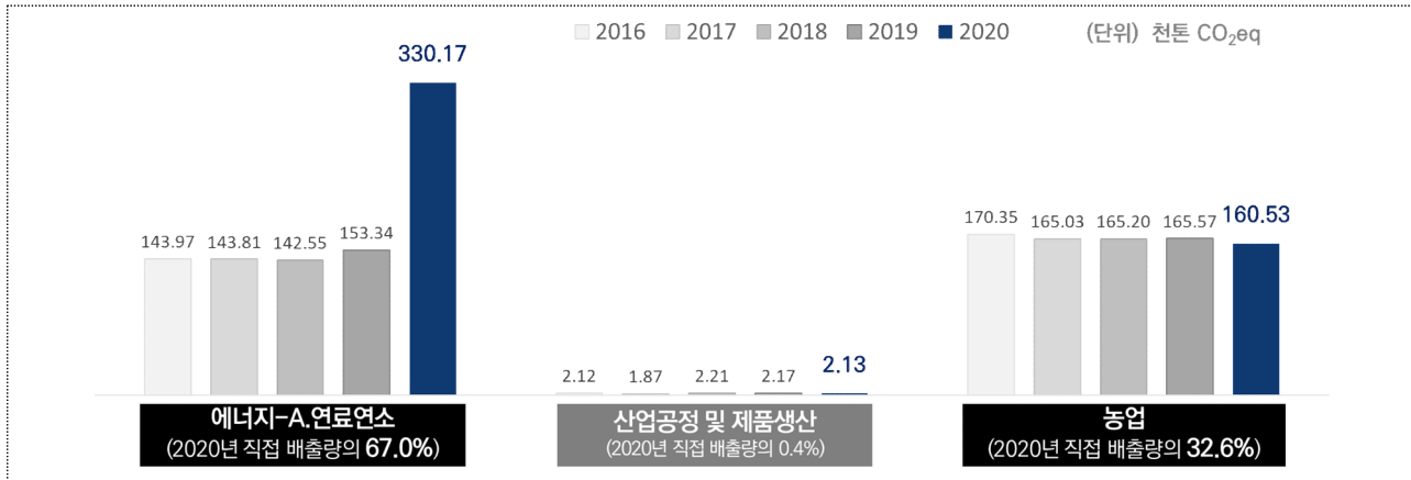
[그림 12] 신안군 온실가스 직접배출량 부문별 현황
