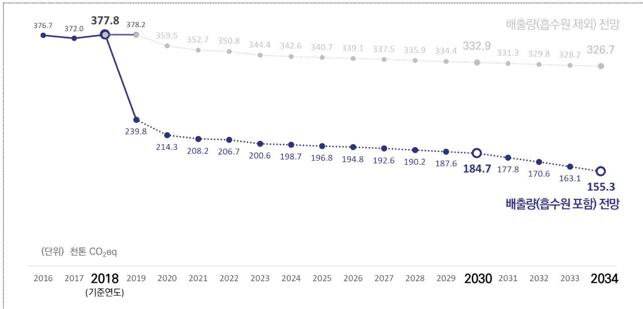
[그림 20] 신안군 온실가스 배출량 전망
