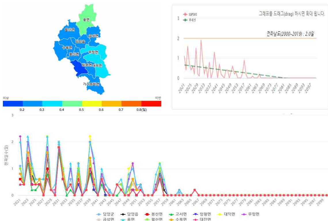
[그림Ⅲ.1 -13] 한파일수, SSP5-8.5, 담양군, 2021~2100년(연별)
