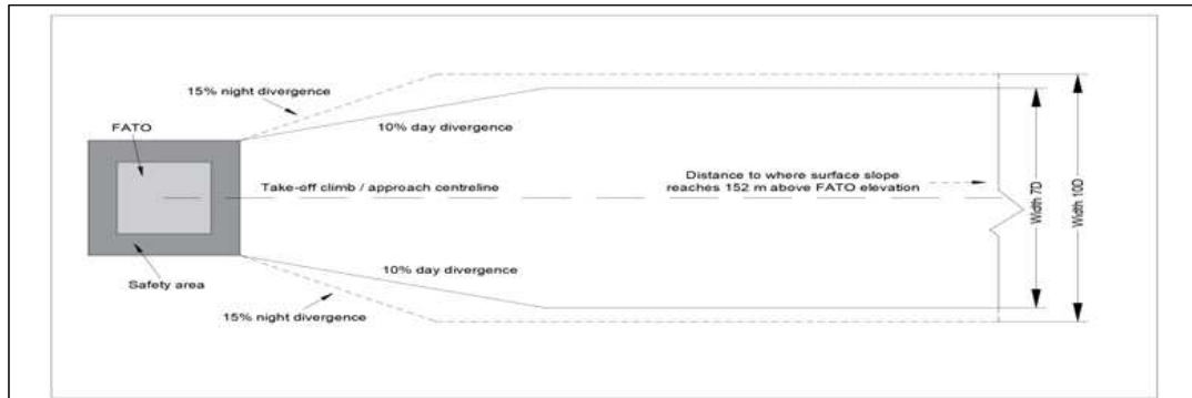
[ UAM 이착륙장 및 안전구역 ]
