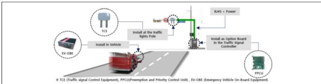
[ 스마트 긴급 차량 우선 신호 개념도 ]
