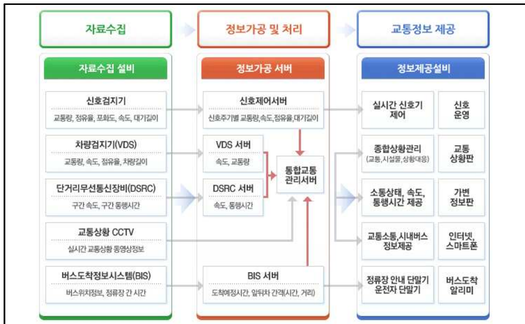
[ 수원시 ITS 구성체계 ]
