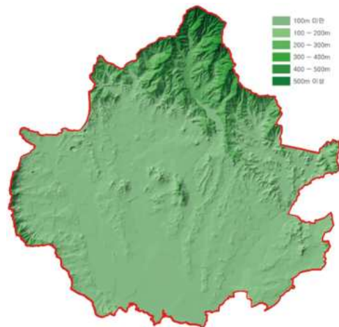
[ 표고분석도 ]
