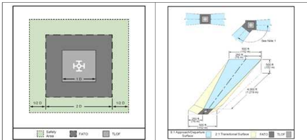
[ UAM 이착륙장 및 안전구역 ]
