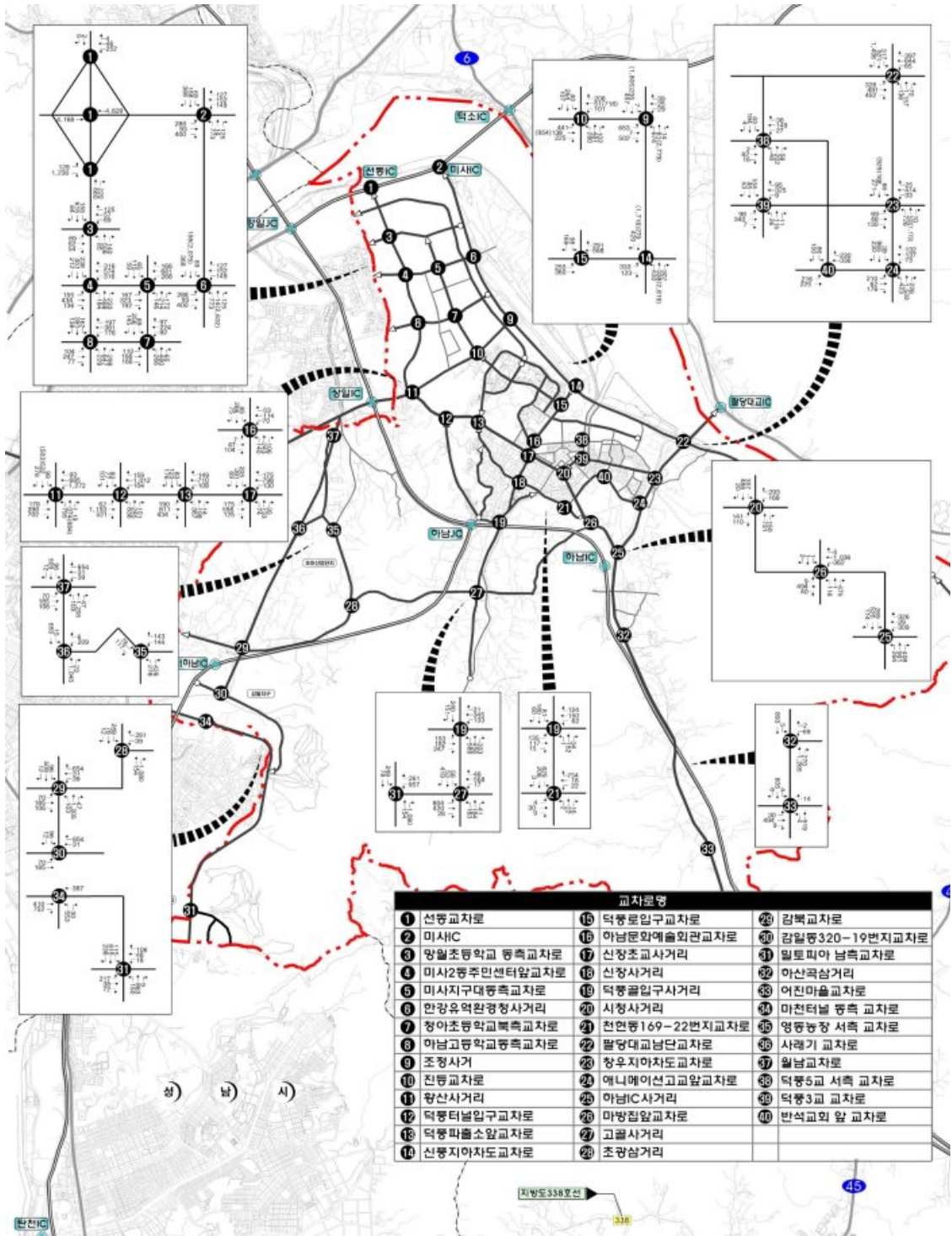
그림Ⅲ.2.6. 교차로교통량 현황도(첨두시 18:00~19:00, PCU/시)
