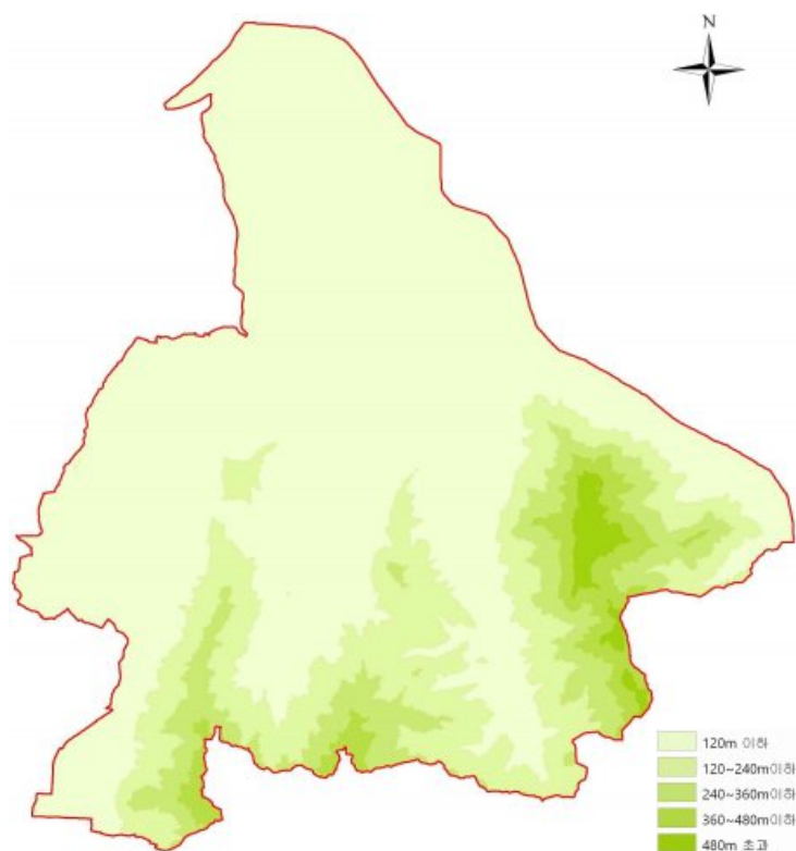
그림 I.2.2. 표고분석도
