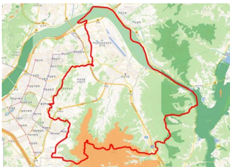
그림Ⅲ.4.5. 생태자연도
