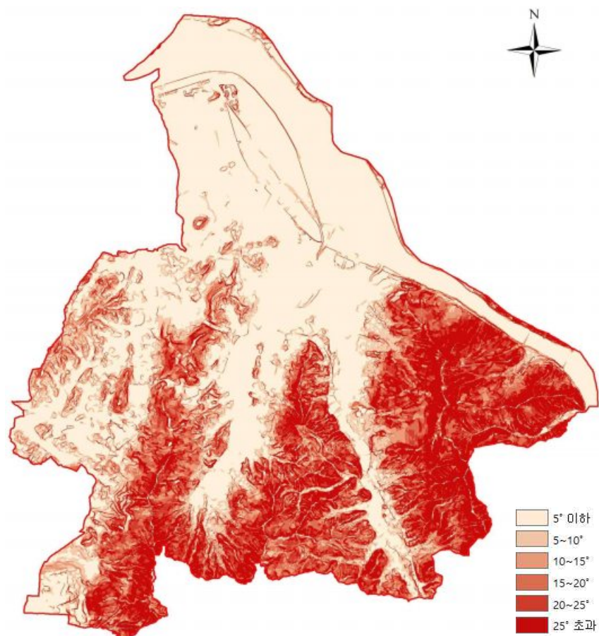
그림 I.2.3. 경사분석도
