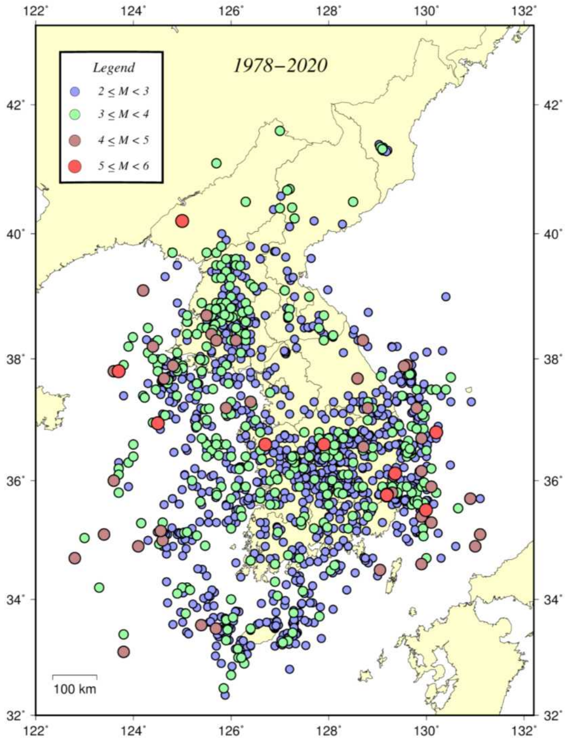
그림 7.2. 진앙분포도(1978년~2020년)
